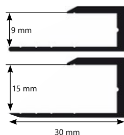
ARRÊT À PARQUET
