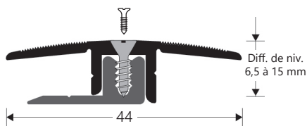
ALU. ANODISÉ 44 mm
