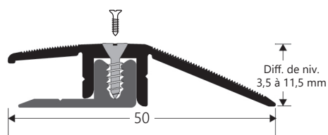
ALU. ANODISÉ 50 mm
